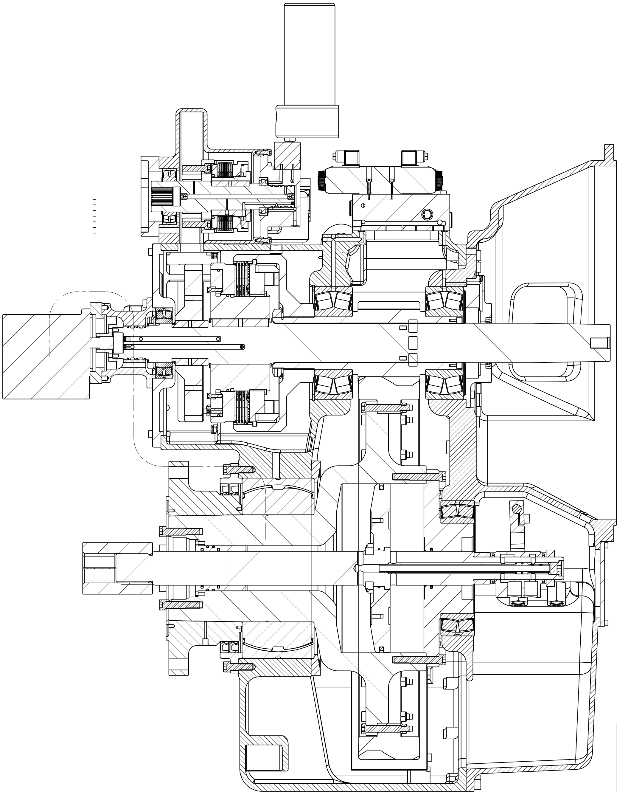
A-A(1:4)
