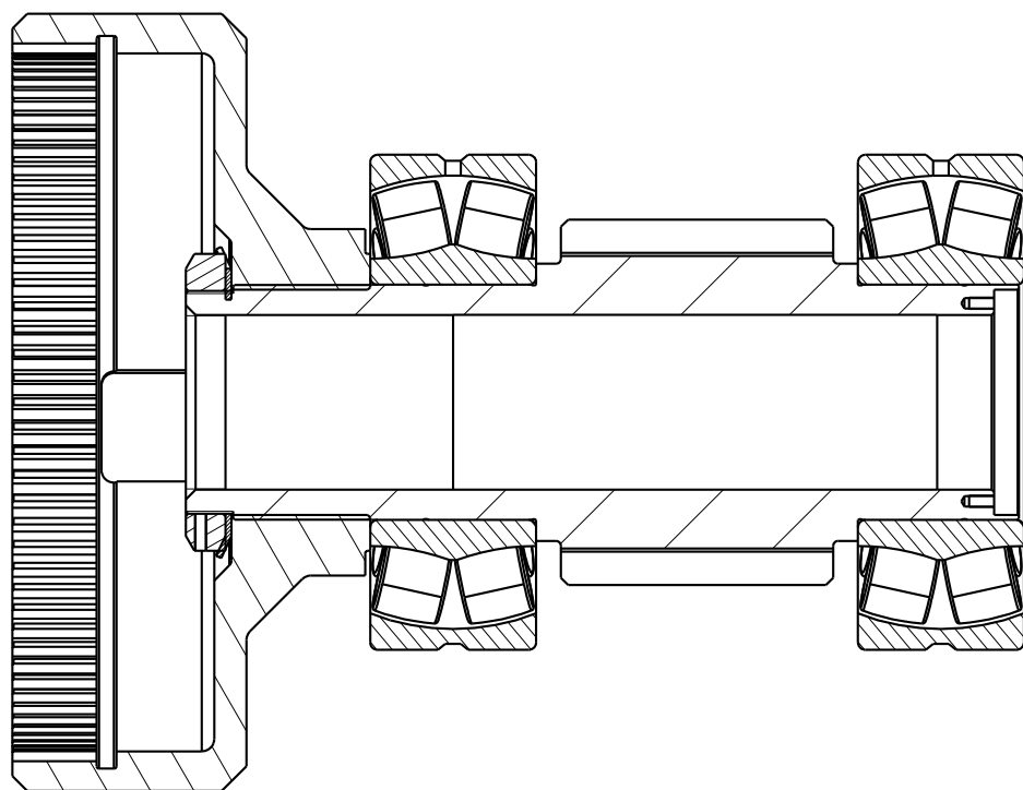
A-A(1:3.333)
