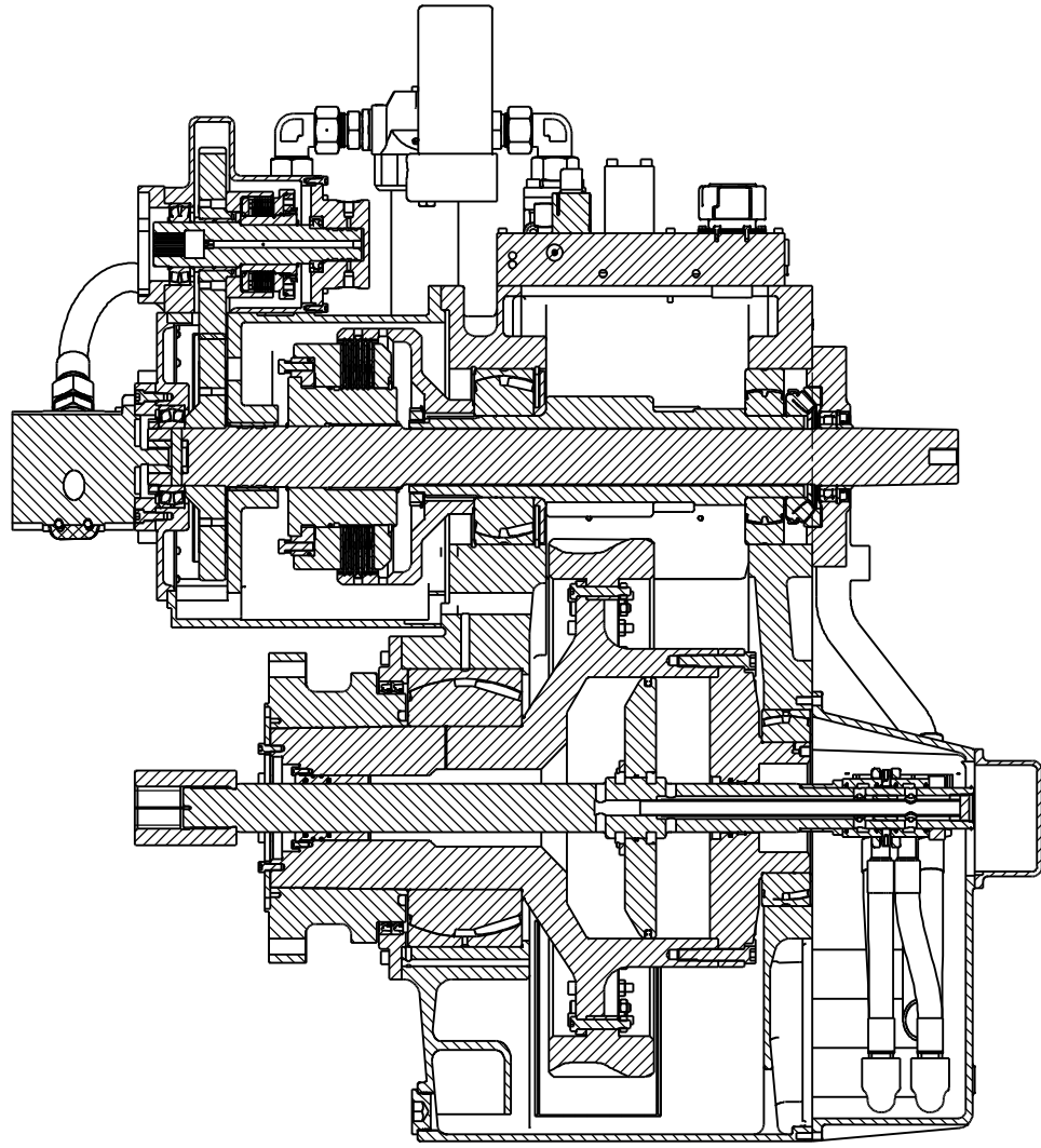
SECTION A-A
