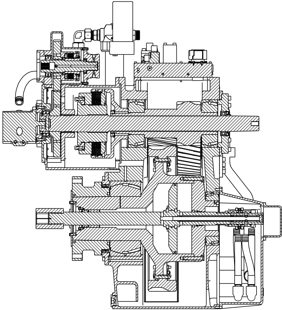
SECTION A-A
