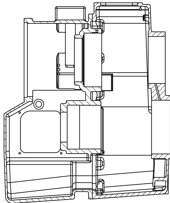
A-A(1:6.667)
