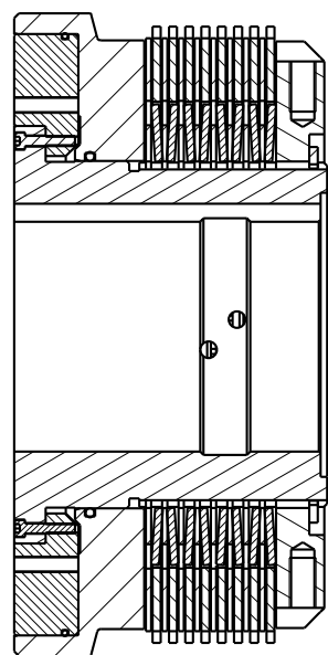
A-A(1:5)
