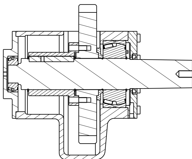
A-A(1:5)
