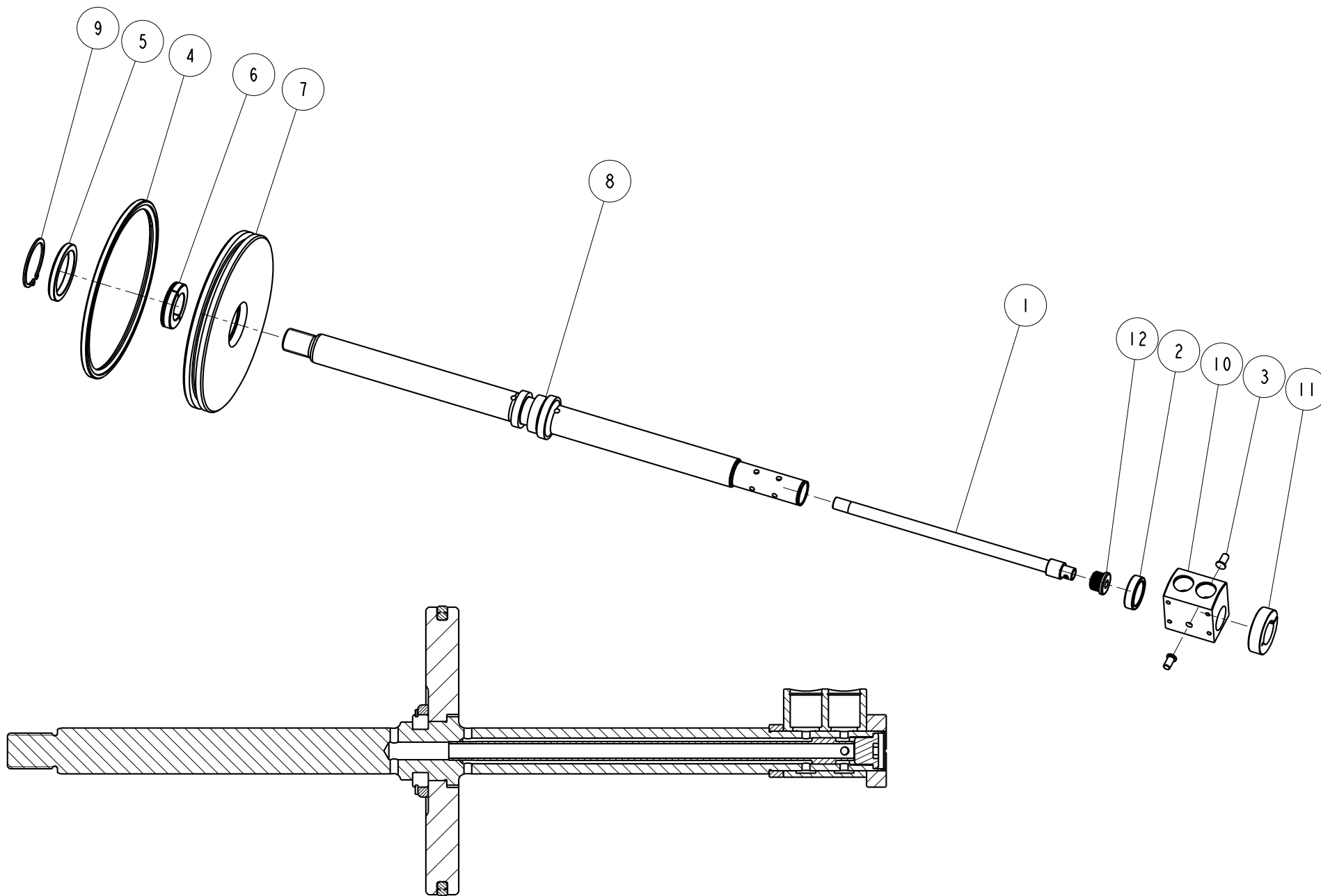
SECTION A-A
